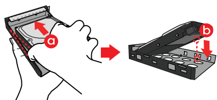
4 - a 트레이에 HDD를 비스듬히 밀어 넣고,
