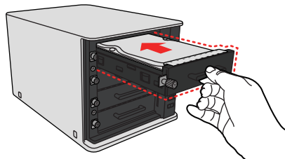
6 HDD가 장착된 트레이를 제품 본체에 밀어넣습니다.
