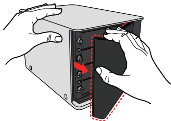
1 제품 전면의 뚜껑을 엽니다.
