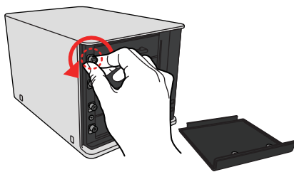
2 트레이 고정나사를 풀니다.
